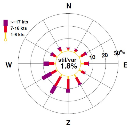
januari, normaal 1991-2020, Schiphol
